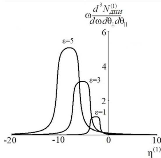
Рис. 5. Спектрально-угловые плотности ДПИ при различных значениях параметра асимметрии \varepsilon . Угол наблюдения: \theta_{\perp} = 2 mrad, \theta_{\parallel} = 0
