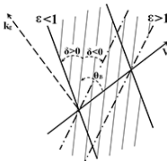
Рис. 2. Асимметричные ( \varepsilon > 1 , \varepsilon < 1 ) отражения излучения от слоистой структуры в геометрии рассеяния Брэгга.
