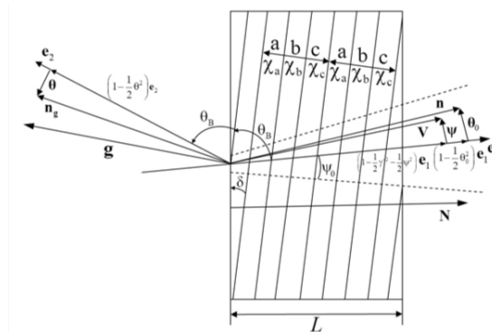
Рис. 1. Геометрия когерентного рентгеновского излучения в многослойной структуре
