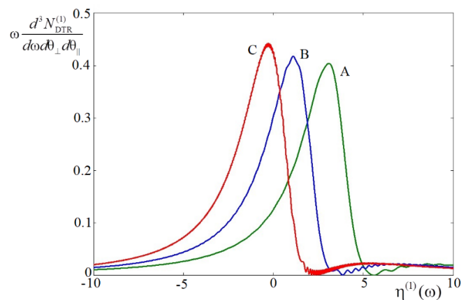
Рис. 7. Спектрально-угловые плотности ДПИ при различных значениях параметра \delta'_a = \chi'_a / \chi' . Обозначения: А ( \delta'_a = 1 ), В ( \delta'_a = 0.5 ), С ( \delta'_a = 0.1 ). Параметры: \delta'_{ab} = 2 , a/b = 0.5 , a/c = 1 , \rho_a = 0.3 , \rho_b = 0.1 , \rho_c = 0.2 , L = 2\mu\text{m} , \varepsilon = 3 , \delta = \pi/40
